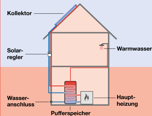
03 Funktionsaufbau solarthermische Anlage
